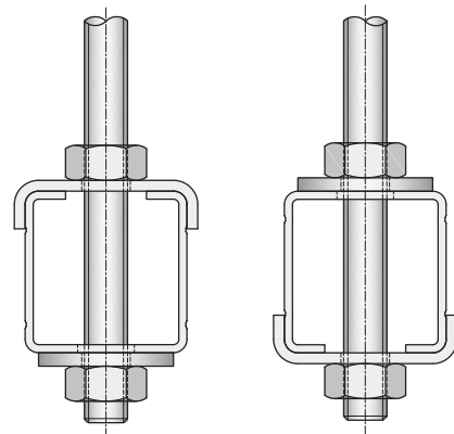
Obrázek 3: Použijte Walraven RapidRail® U-podložku na otevřené straně lišty
