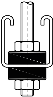
RapidStrut®
